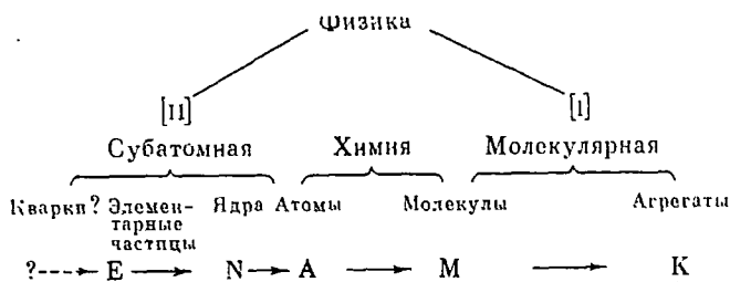
Р и с. 1. «Раздвоение» современной физики
