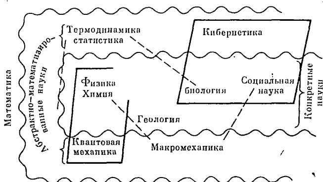
Р и с. 5 «Раздвоение» наук по степени их абстрактности
