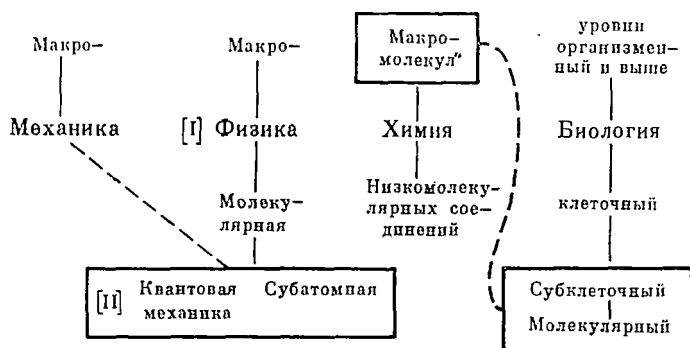
Р и с. 3. «Раздвоение» наук по масштабам (уровням) их объектов
